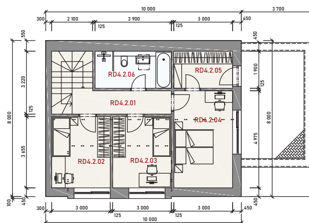
PÔDORYS PODKROVIA
