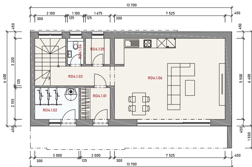
PÔDORYS PRÍZEMIA
